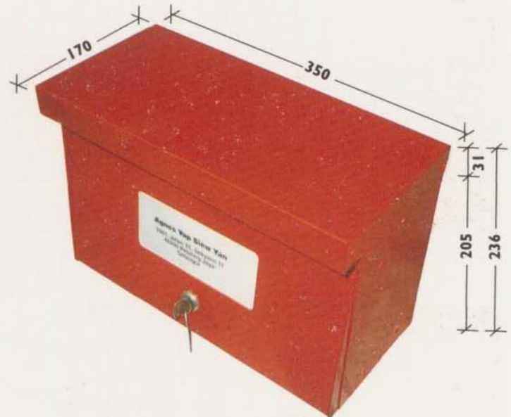
TYPE : SU 350 (W) x 236 (H) x 170 (D) DESIGN : TOP HUNG WITH WINDOW DISPLAY
