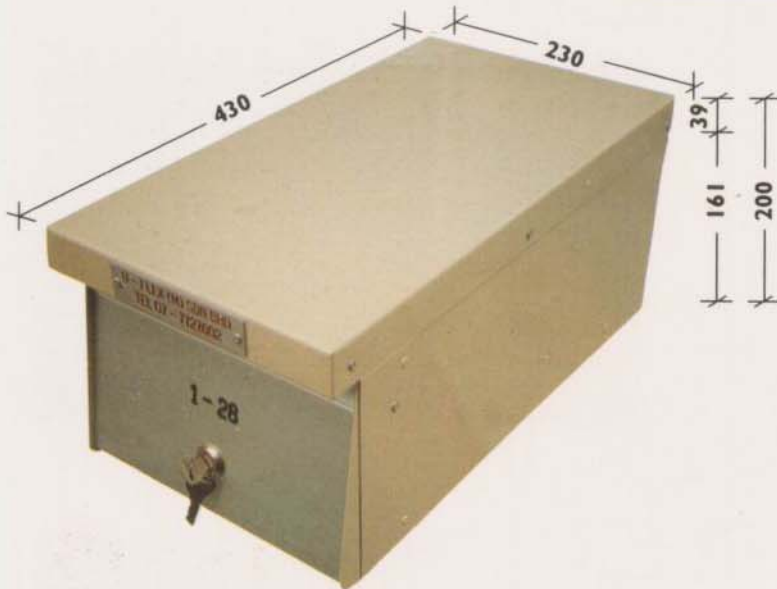
TYPE : LC 230 (W) x 200 (H) x 430 (D) DESIGN : TOP HUNG PLAIN DOOR
